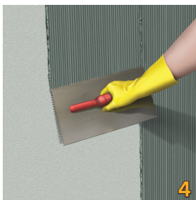
Thi công lớp thứ nhất theo phương dọc bằng chổi, cọ quét hay bay thép.
