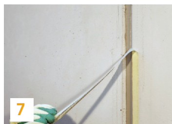
7 Gỡ bỏ băng keo viền mỗi nối
